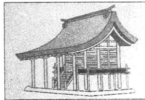
流れ造り
