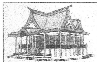
権現造り
