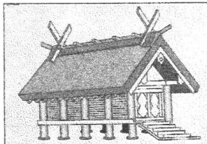
住吉造り
