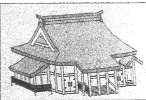
祇園造り
